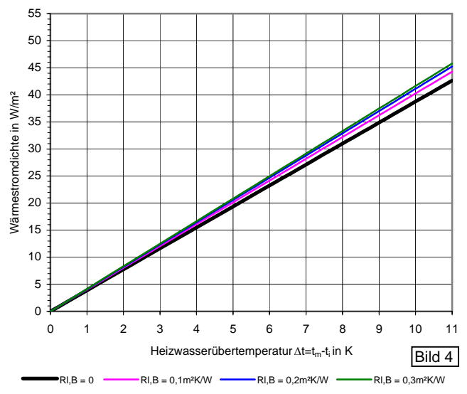
Stationäre Heizleistung der Decke
