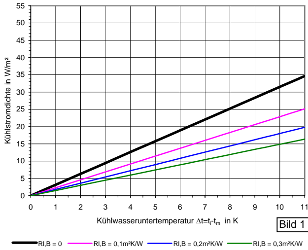
Stationäre Kühlleistung des Fußbodens
