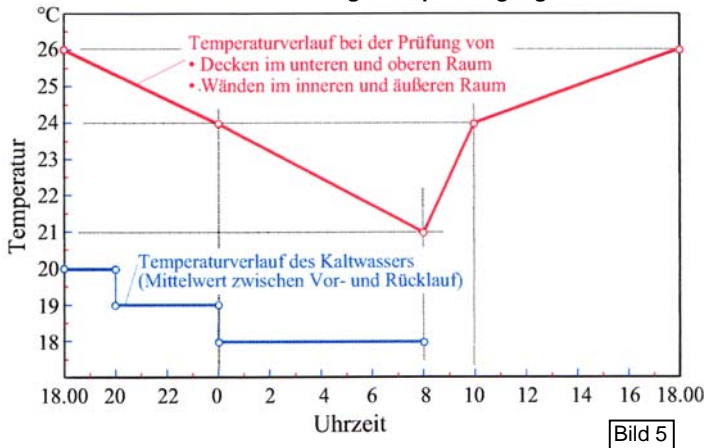
Der instationären Leistungsermittlung zugrundegelegte Referenz-Tagestemperaturgang
