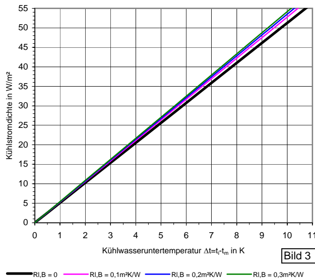
Stationäre Kühlleistung der Decke
