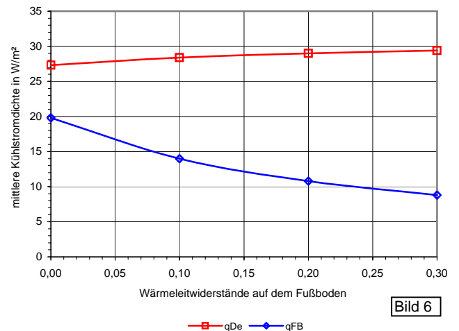
Mittlere instationäre Kühlleistung zur Hauptnutzungszeit
