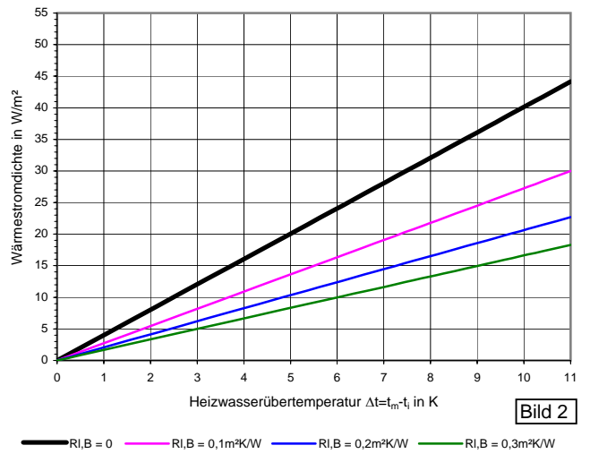
Stationäre Heizleistung des Fußbodens
